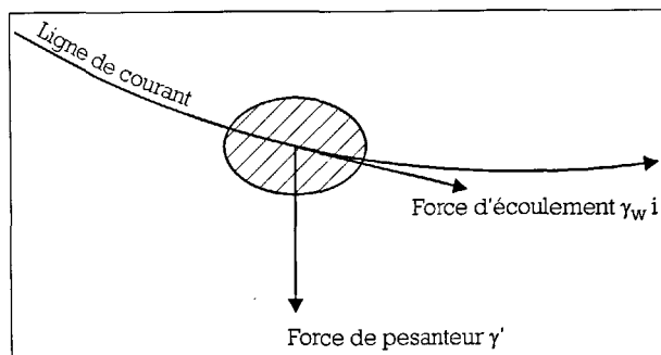
Figure 4 - Forces appliquées à un grain de sol.
