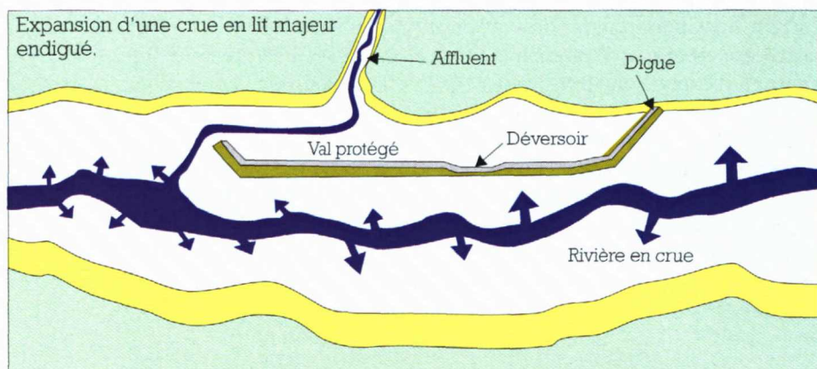
Figure 3.a : Expansion d'une crue en lit majeur endigué.
