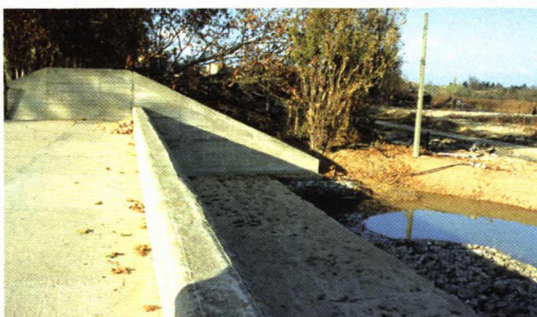
Photo 3.5 – Déversoir de Sallèdles d'Aude après la crue des 12-13/11/1999 : dégradations sur le radier parafouille en gabions.
