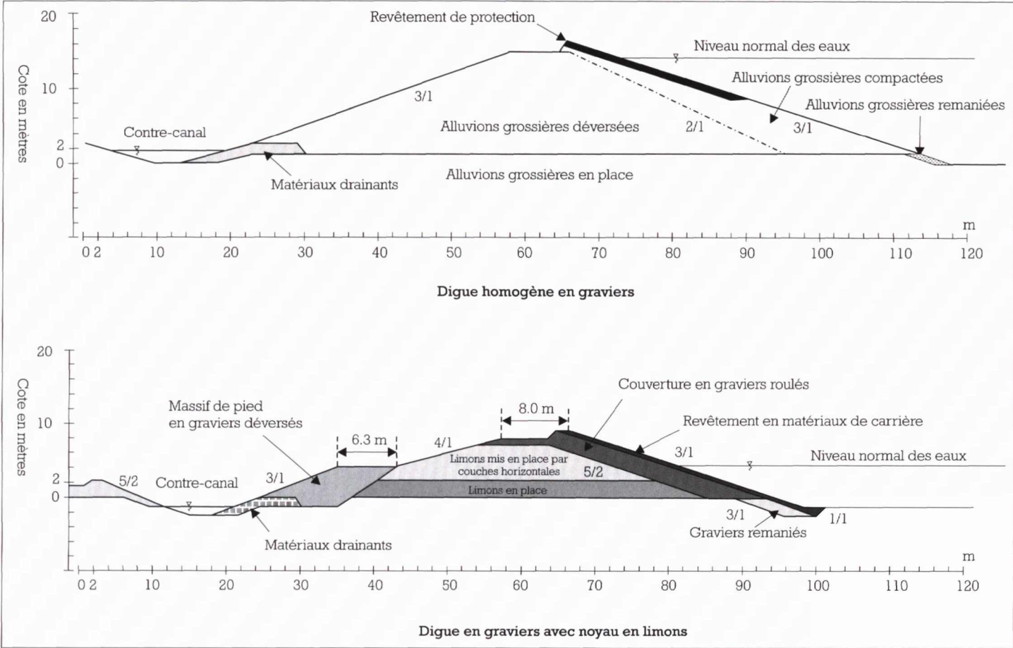
Figures 6 : Coupes types des digues du Rhône dans le secteur aménagé par CNR.
