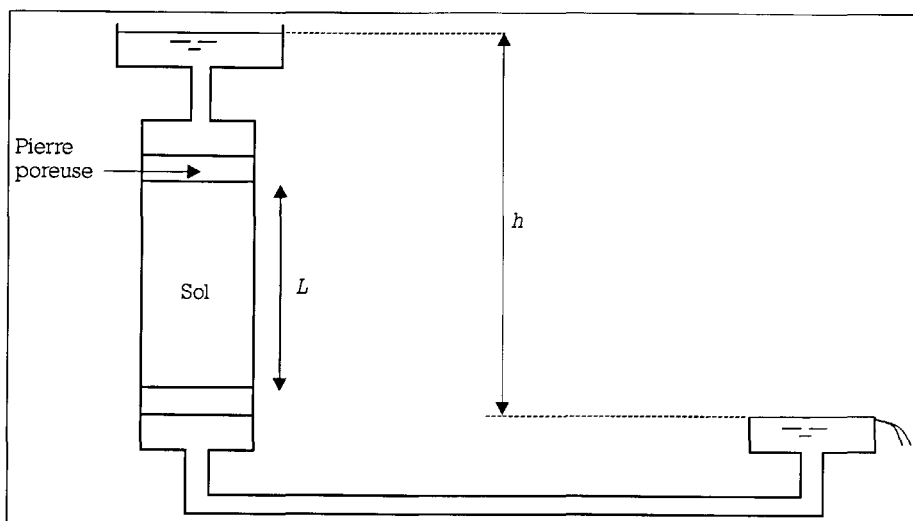
Figure 1 - Principe du perméamètre : échantillon de sol soumis à un gradient hydraulique i = h/L .
