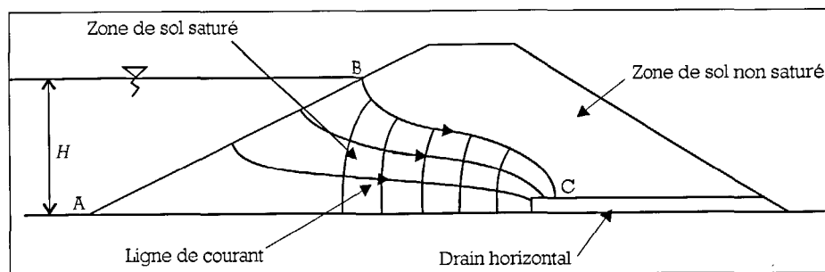
Figure 3 - Saturation d'un ouvrage hydraulique en terre.
