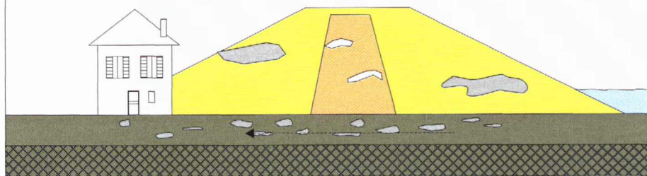
Figures 11 : Mécanisme du renard hydraulique.
