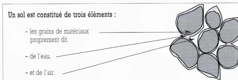
Figure 1 - Constitution d'un sol.
