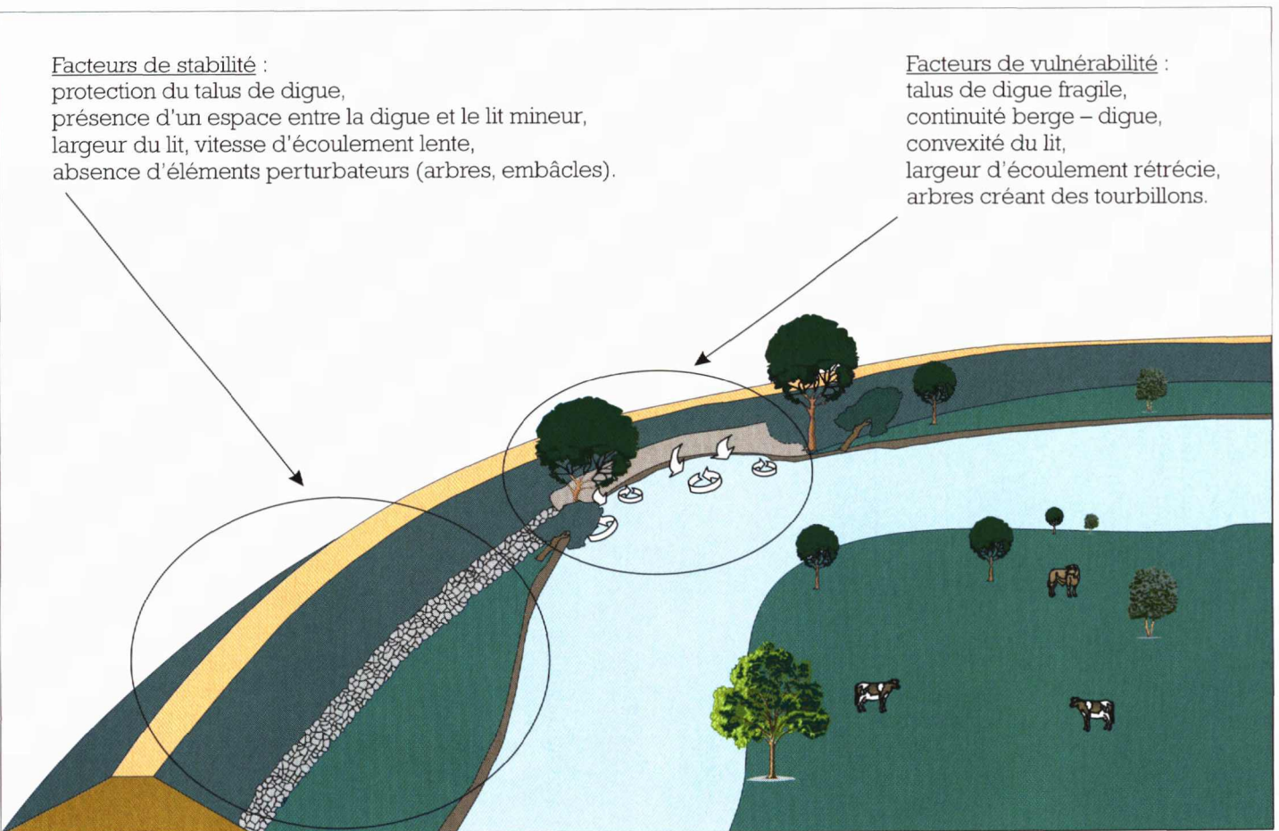
Figures 10 : Mécanisme de l'affouillement en pied de digue.
