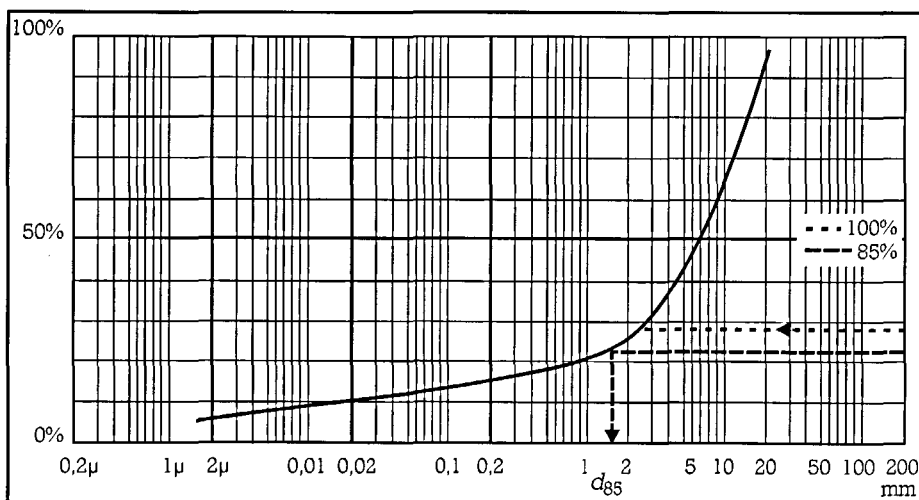
Figure 7 - Cas d'un sol à granulométrie discontinue.
