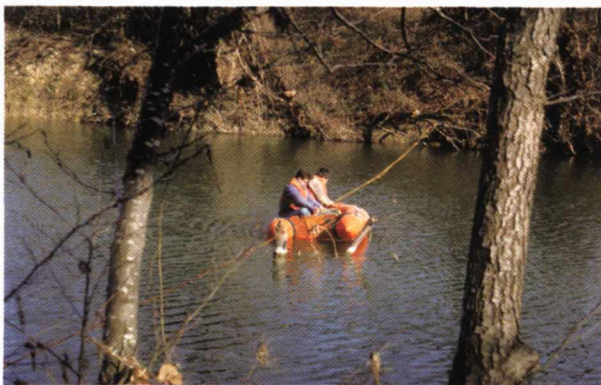
Photo 6.2 – Relevé bathymétrique au décimètre plombé sur un profil en travers du Vidourle dans sa partie endiguée.
