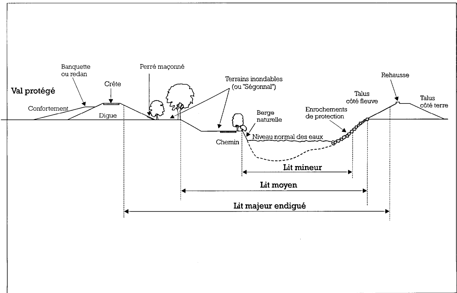
Figure 1 : Coupe-type d'une vallée endiguée.
