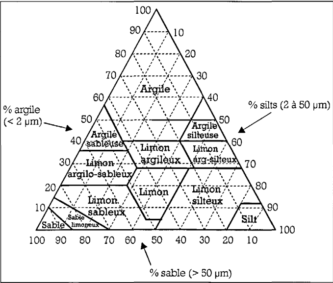
Figure 6 - Classification triangulaire des sols fins.
