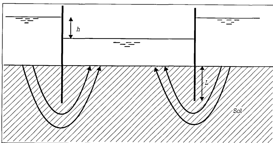
Figure 5 - Écoulement sous une enceinte en palplanches.
