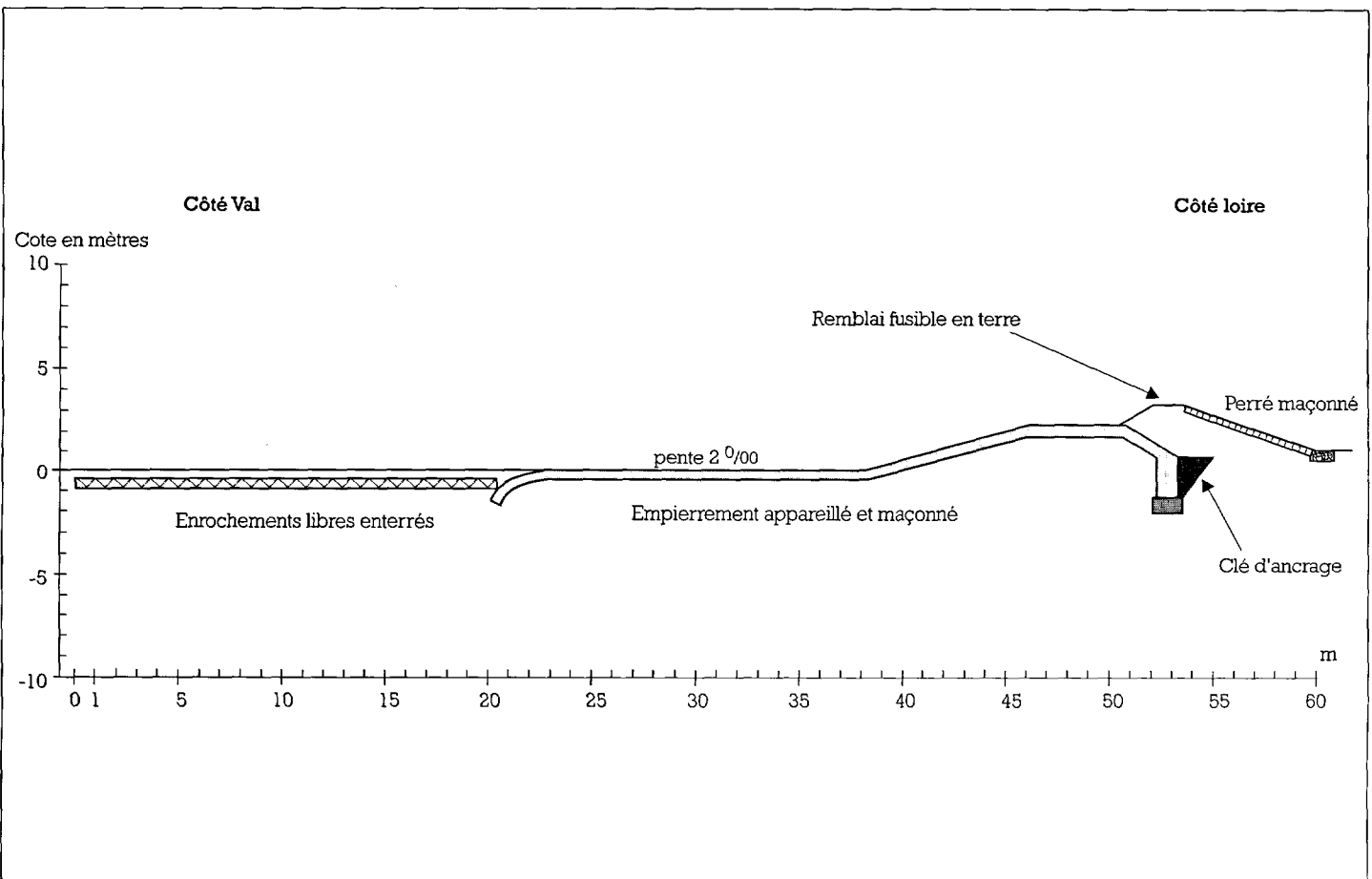
Figure 8 : Coupe type d'un dépenseur Conroy sur la Loire (Ouzouer).
