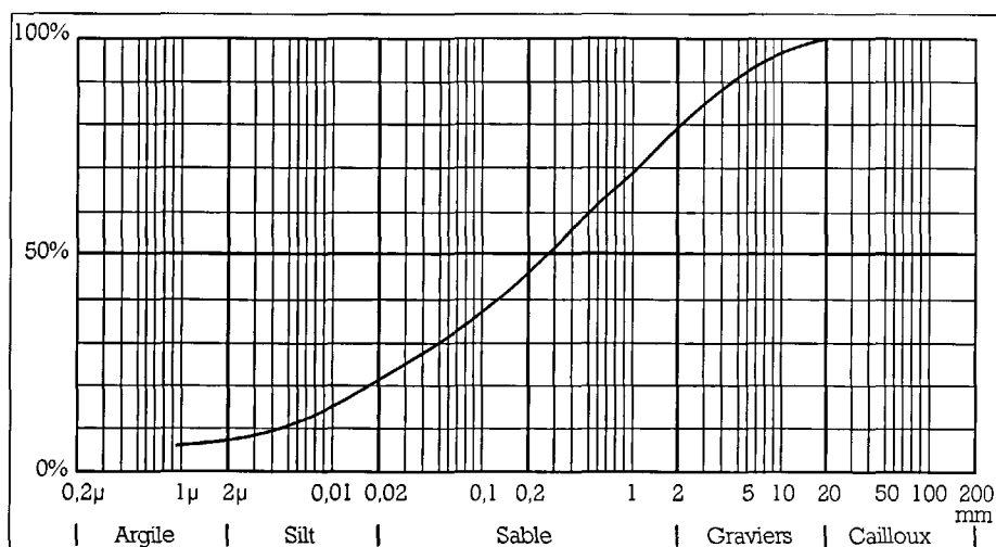
Figure 2 - Courbe granulométrique.
