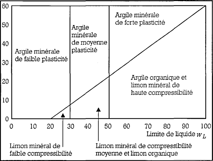
Figure 5 - Abaque de plasticité de Casagrande.
