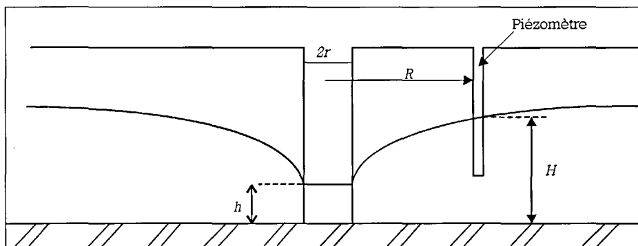
Figure 6 - Rabattement d'une nappe.
