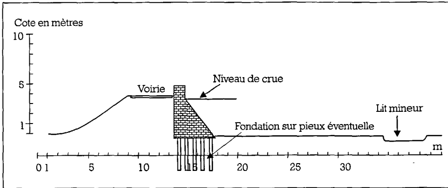
Figure 7 : Coupe type d'une digue en maçonnerie.
