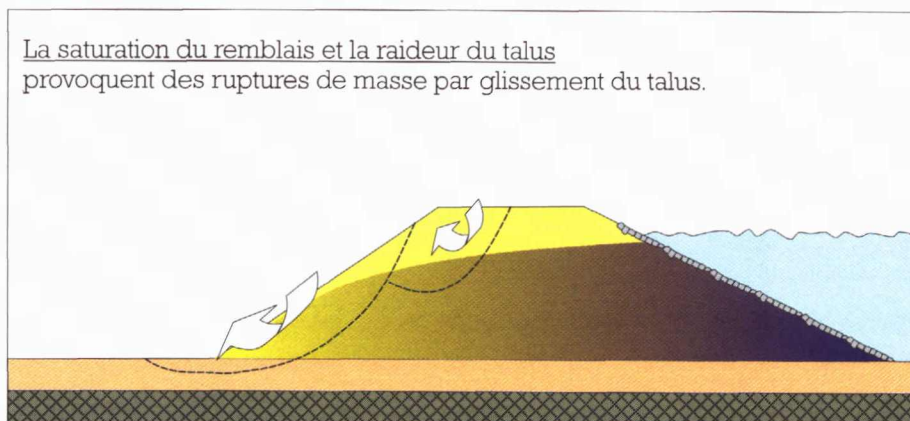
Figure 12 - 1 Mécanisme de rupture du talus aval (côté terre) en situation de crue.
